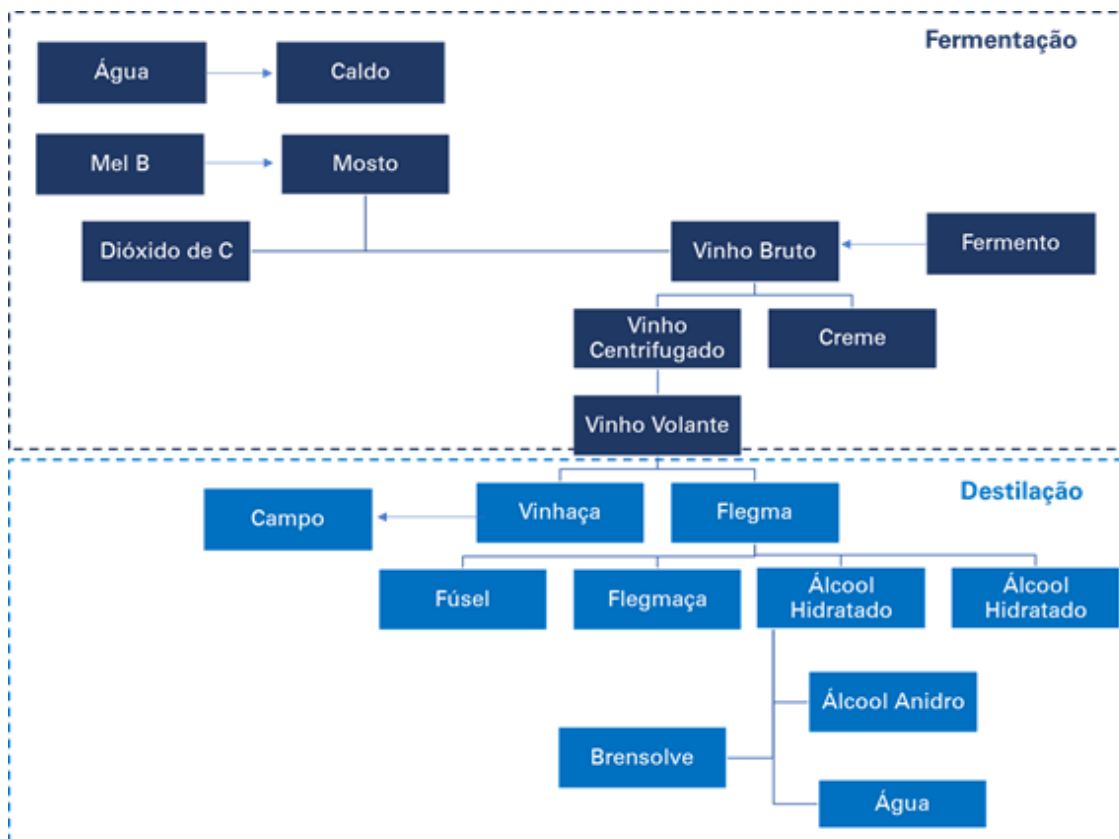
Figura 2: Fluxograma de Processo – Usina Bazan.
