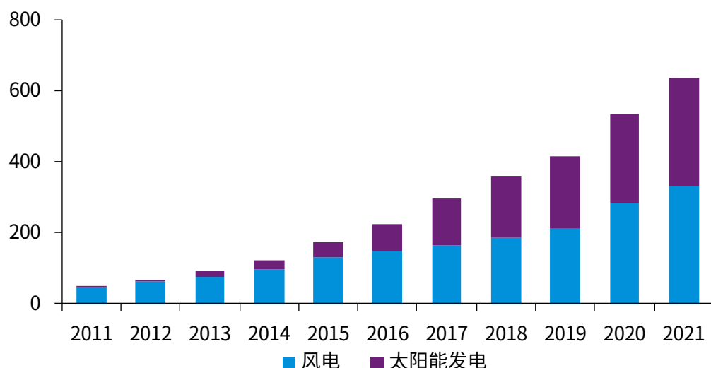
图18 风电、太阳能发电装机容量，百万千瓦
