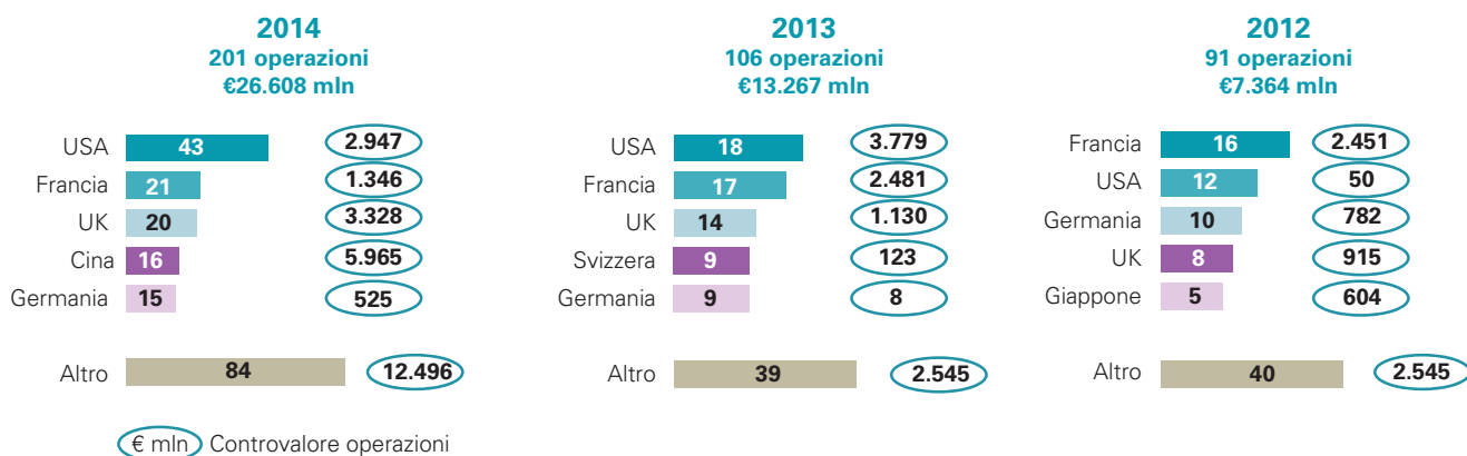
Grafico 23 – Operazioni Estero su Italia 2012-2014: i principali Paesi acquirenti
