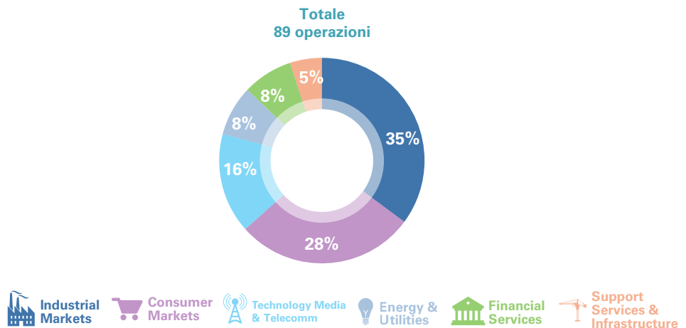
Grafico 25 – Operazioni Italia su Estero: breakdown per macro settore della società acquisita (target)
